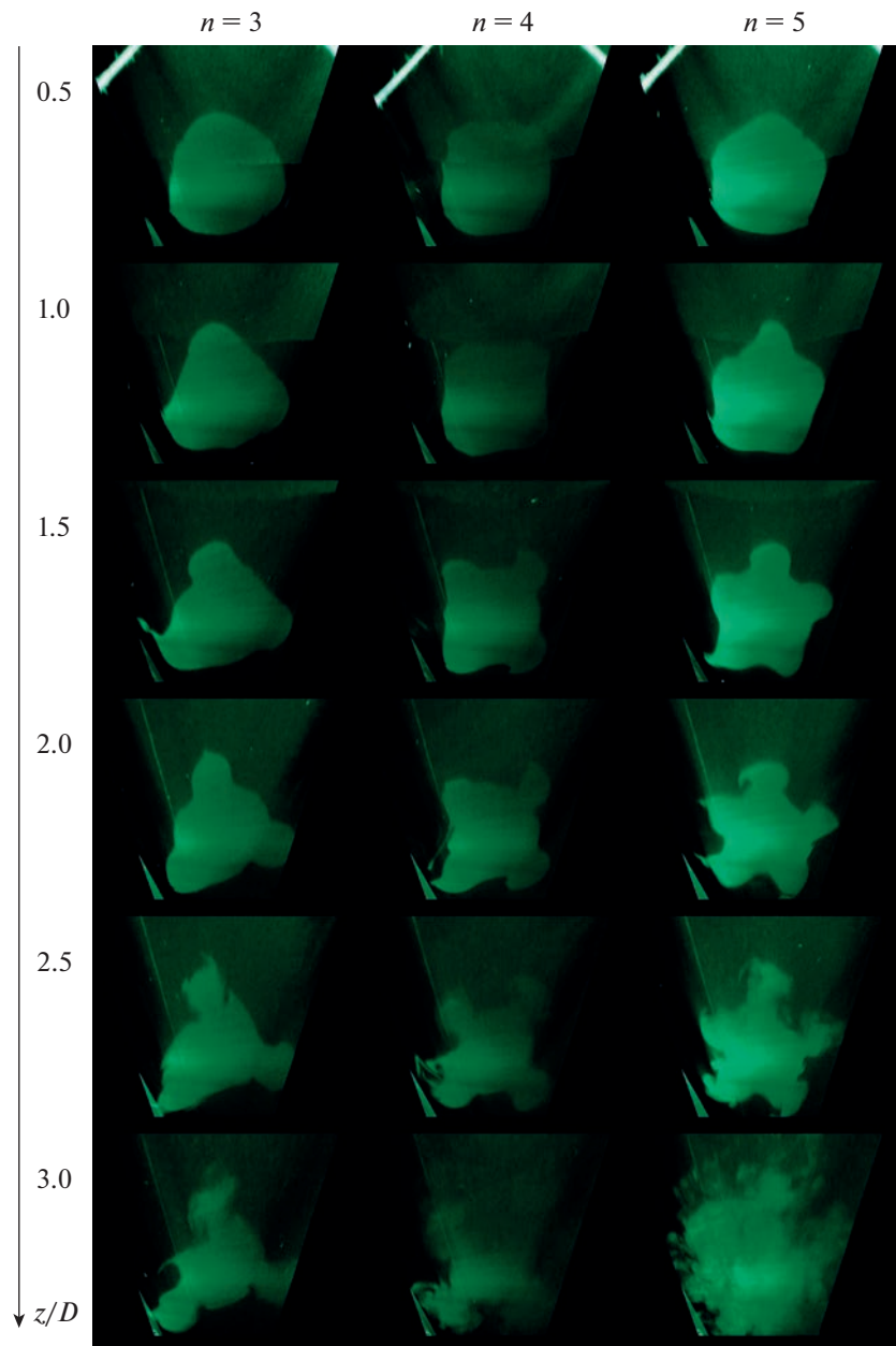
Рис. 6. Эволюция стационарных возмущений, вносимых дефлекторами с азимутальными числами n = 3, 4, 5 и \epsilon = 0.1 в фотографиях поперечного среза.
